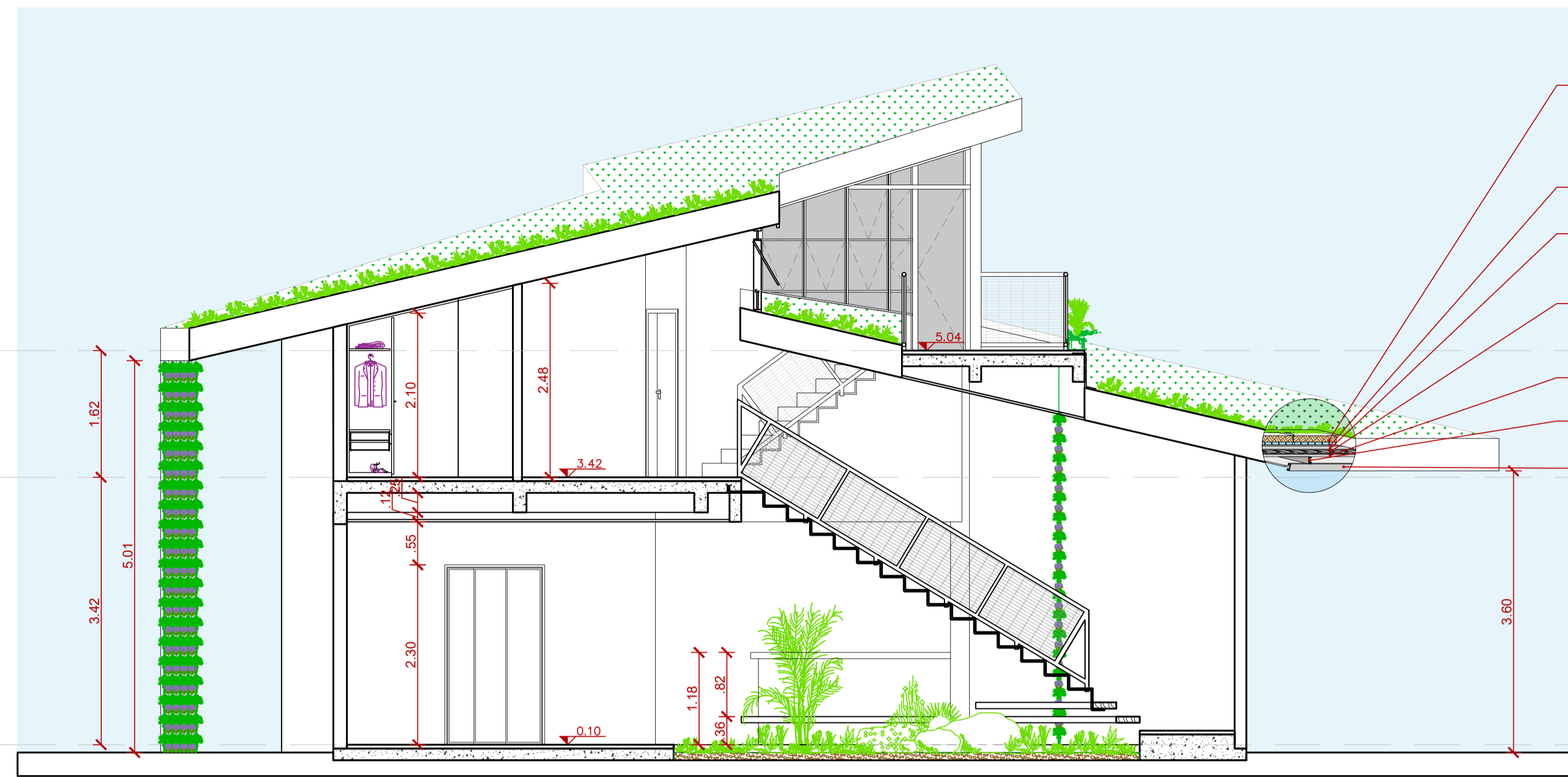
05 CORTE ESCALA: 1/50
