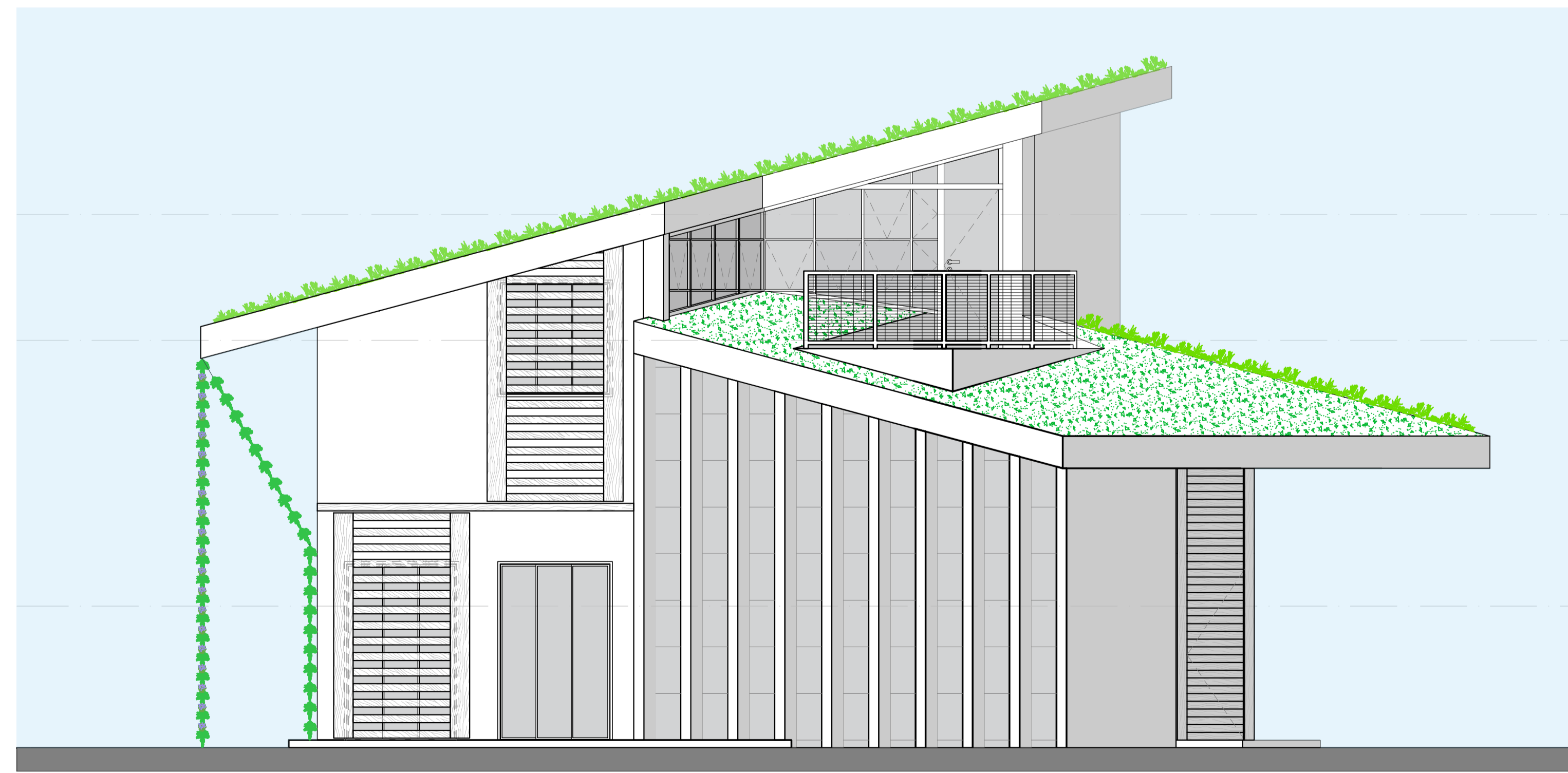
06 FACHADA SU-SUDESTE ESCALA: 1/50
